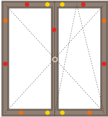
Schéma de principe selon dimensions
